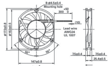
UF-DA1725B24H Ölçü : 172 x 147 x 25mm
