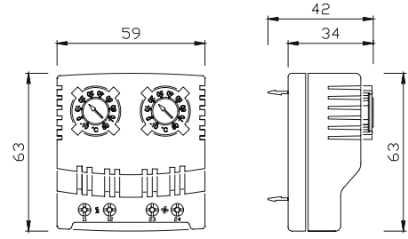
QHT NCNO : Double Termostat
