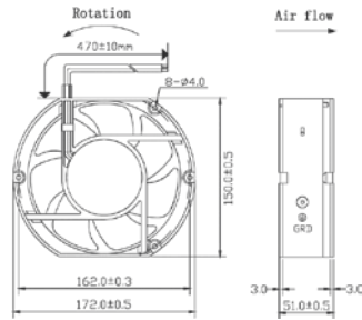
UF-DA1751B24H Ölçü : 172 x 150 x 51mm
